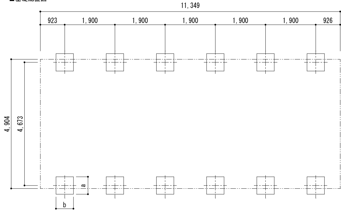
■基礎配置図
